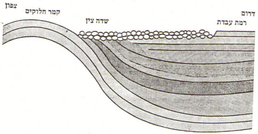
שלב ב' - אמצע נאוגן - נחלים רחבים זורמים באיזור שדה ציץ
