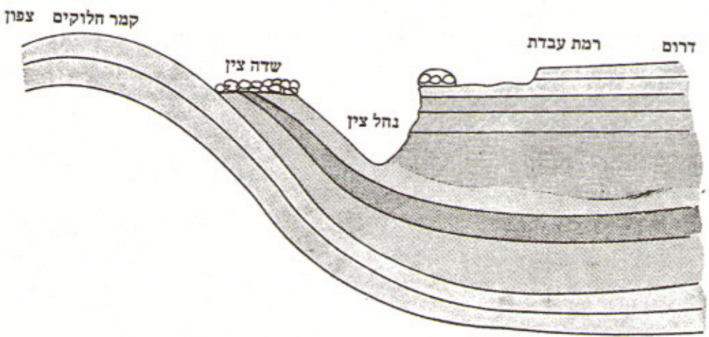
שלב ג' - כיום - נחל ציץ מחותר עמוק מתחת לקונגלומרט הנאוגני
